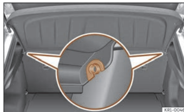
Fig. 166 În portbagaj: demontarea și montarea raftului depozitare spate.
