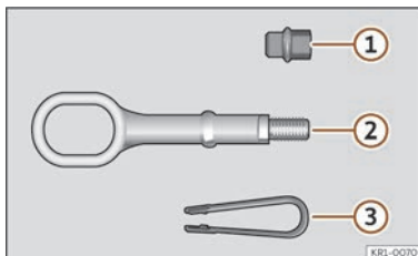
Fig. 181 Sub podeaua portbagajului: trusa de scule.
