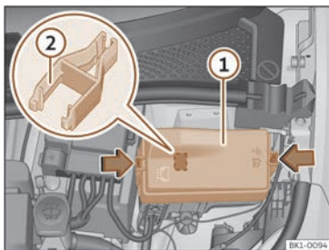
Fig. 193 În compartimentul motor: capacul cutiei cu siguranțe.
