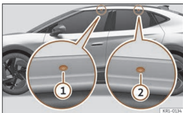
Fig. 174 Punctele de prindere pentru barele transversale pentru suportul pentru portbagajul de acoperiș.
