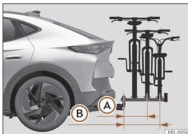
Fig. 178 Reprezentare schematică a ieșirii maxime în consolă a unui suport de biciclete pentru două sau trei biciclete.
