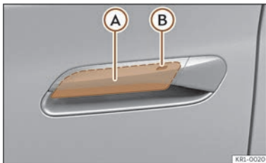
Fig. 69 Mânerul ușii: suprafețele senzorilor.
