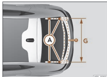
Fig. 180 Dispozitiv de remorcă: dimensiuni și puncte de fixare.
