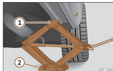
Fig. 208 Traversa: montarea cricului pe autovehicul.
