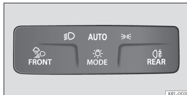
Fig. 93 Panoul de bord: panoul pentru lumini.
