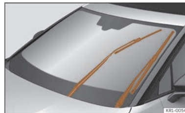
Fig. 182 Ștergătoarele în poziția de service.
