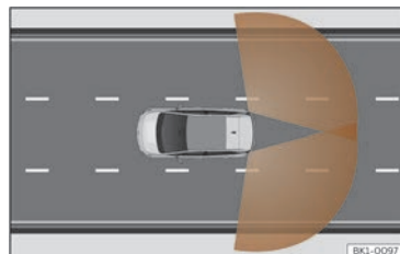
Fig. 116 Zone de detecție senzori.
