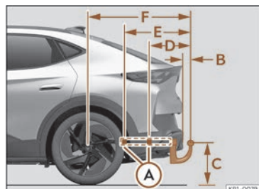
Fig. 179 Dispozitiv de remorcă: dimensiuni și puncte de fixare.
