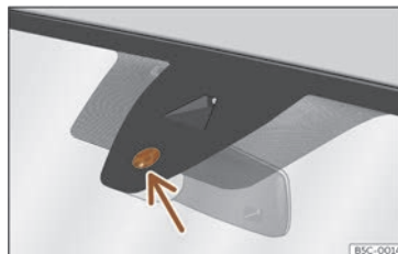
Fig. 106 Senzorul de temperatură și umiditate a parbrizului.
