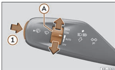
Fig. 97 Acționare ștergătoare.
