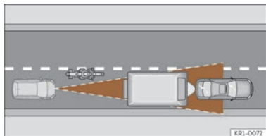
Fig. 125 Motociclist în față, în afara razei de acțiune a senzorului cu radar.
